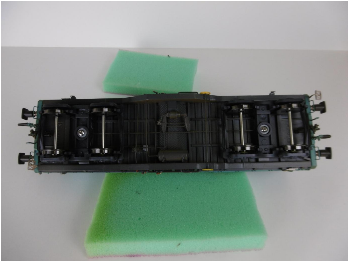
Foto 1b Ansicht detaillierte Bremsanlage
